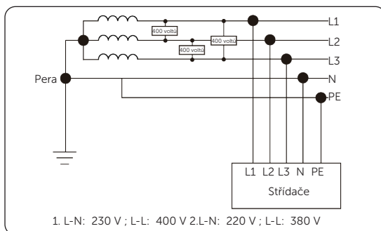
Obrázky- 24 Podporované sítě: TN-C-S
