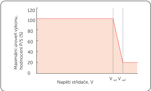
Obrázky- 107 P(u) křivka
