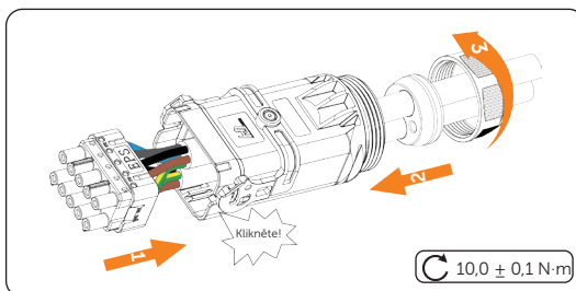
Obrázky- 818 Montáž AC konekturů
