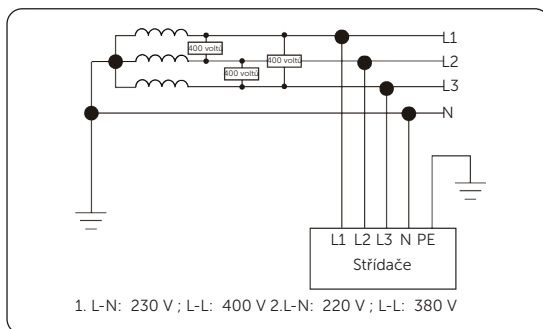
Obrázky- 22 Podporované sítě: TT
