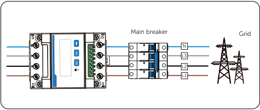
Obrázky- 1528 Připojení přímého měřiče k elektrické síti
