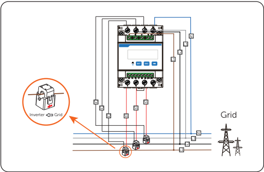
Obrazky- 1532 Připojení CT připojených měřičů k elektrické síti
