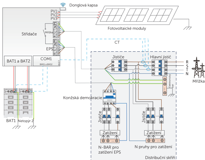
Obrázky- 26 Domácí zálohování v části Evropy
